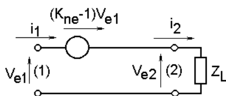
Рис. 2. Эквивалентная схема КОСН
