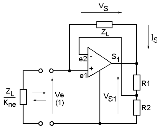
Рис. 3. Схема КОСН с незаземленной нагрузкой
