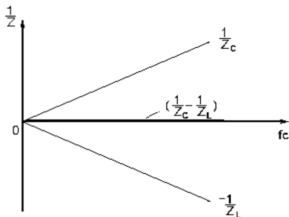
Рис. 5. Результирующая зависимость емкости сети и проводимости КОСН от частоты
