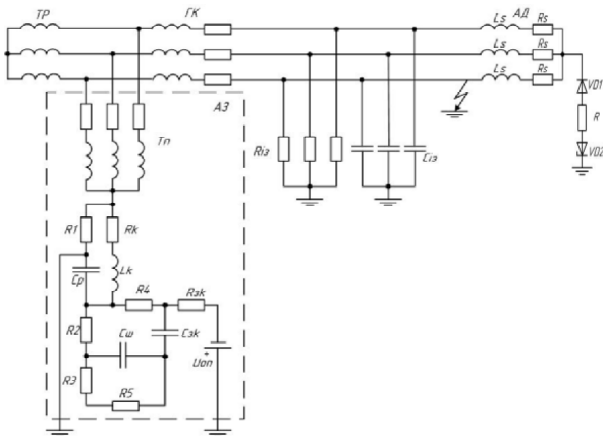
Рис. 2. Схема електротехнічного комплексу дільниці шахти в стані однофазного замикання на землю з урахуванням наявності апарата захисту АЗУР-4
