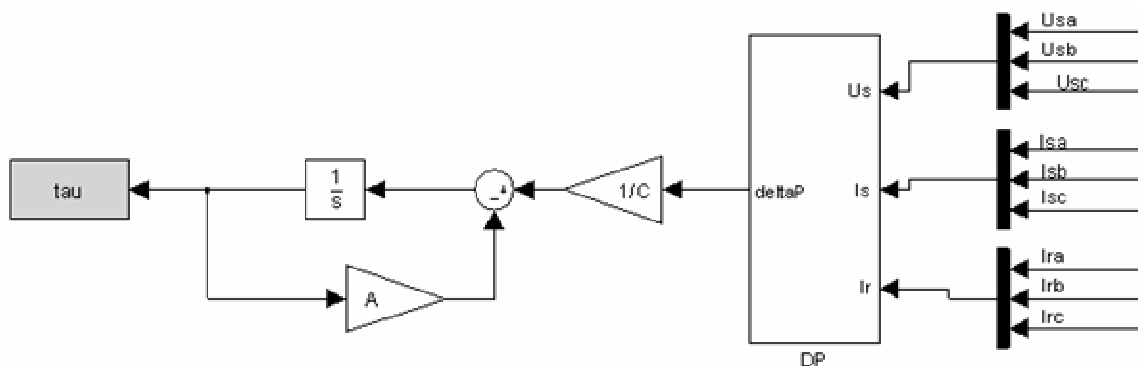
Рис. 1. Тепловая модель асинхронного двигателя
