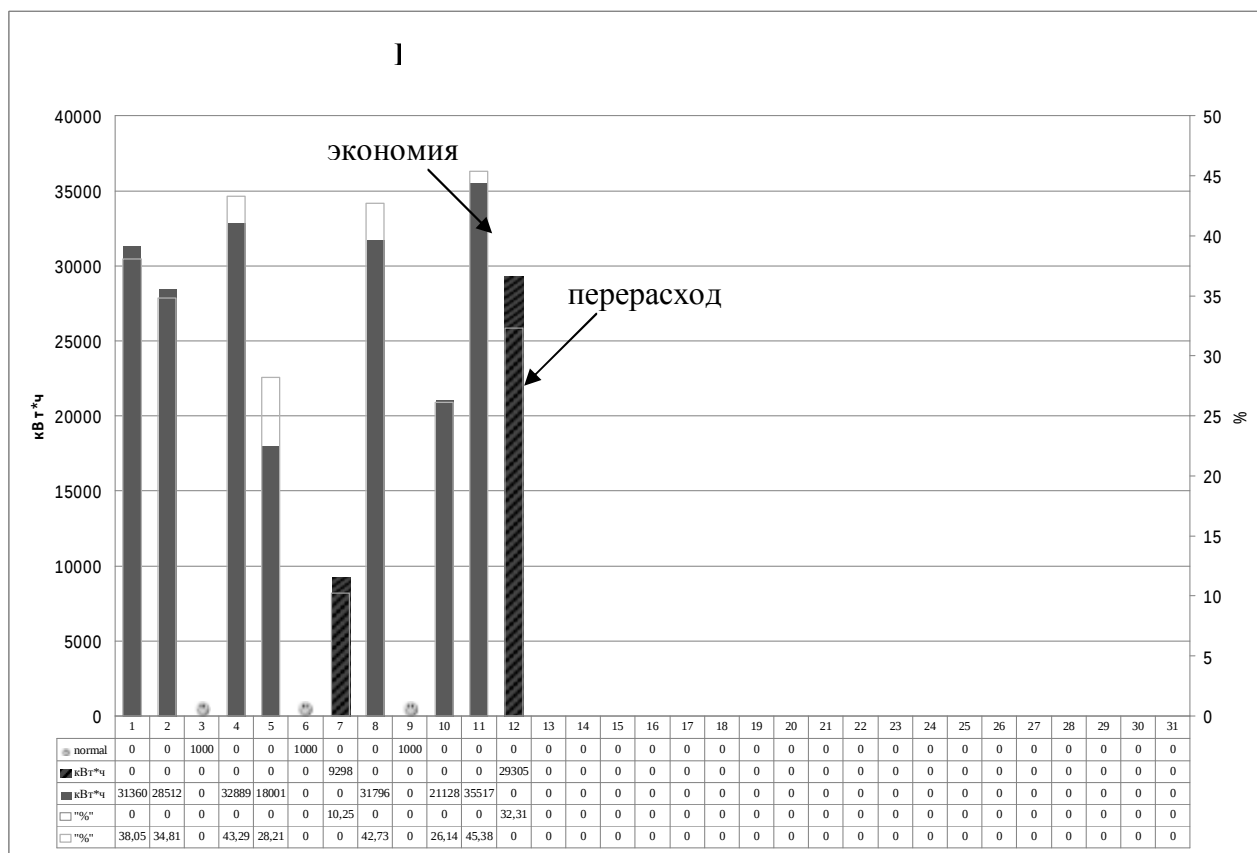
Рис.2. Результаты контроля энергоэффективности шахты Героев Космоса
